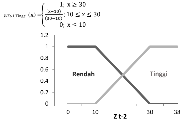
Gambar 2 FungsiKeanggotaan Input Zt-2
